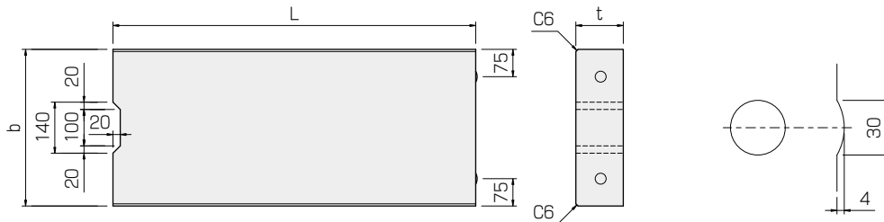
突起部詳細図
