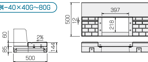
管理樹 M樹-30×30G~80G
