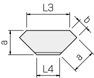
3号ブロック
