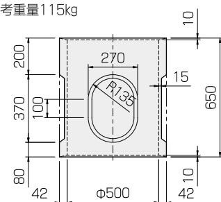
側塊B
