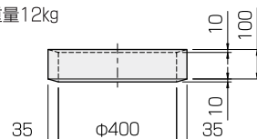
側塊C
