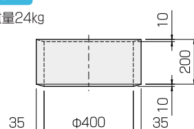
側塊D
