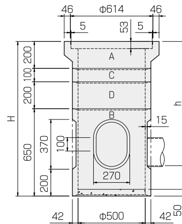
雨水桷(RB型)
