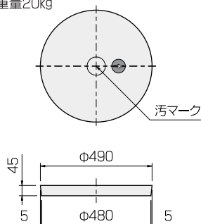
汚水枳蓋
