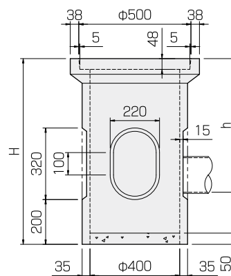
雨水枳(RA型)
