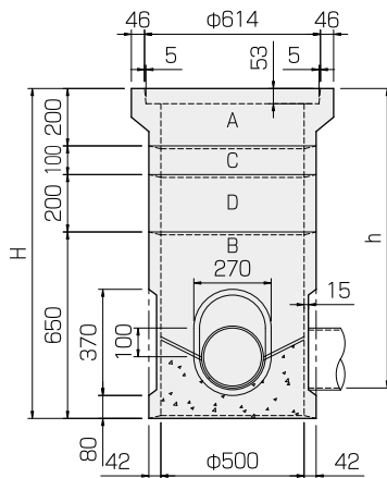
污水桷(SB型)
