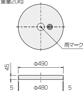
雨水枳蓋
