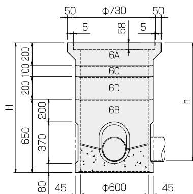
汚水樹(SC型)
