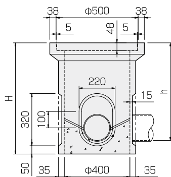
汚水枳(SA型)
