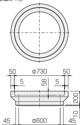
側塊6A
