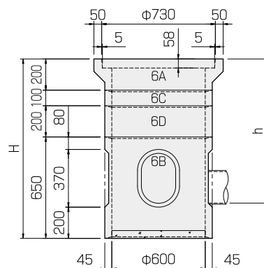
雨水樹(RC型)
