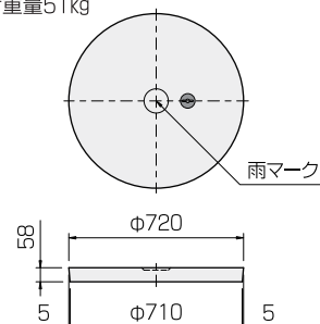
雨水樹蓋
