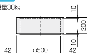
側塊D
