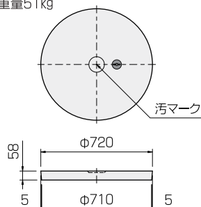
汚水樹蓋
