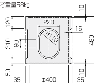
側塊B
