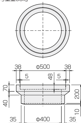
側塊A
