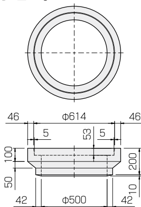
側塊A
