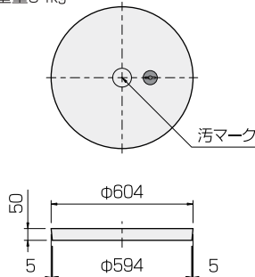
污水桷蓋
