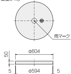
雨水桷蓋
