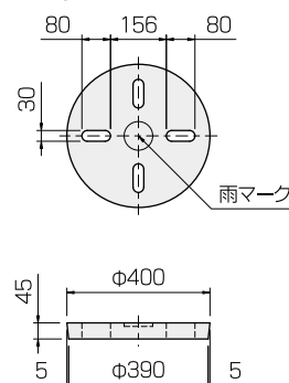
雨水枡蓋
