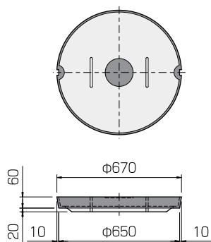
汚水樹蓋
