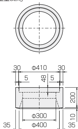
側塊A
