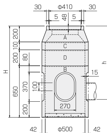
雨水枡(TMR50)
