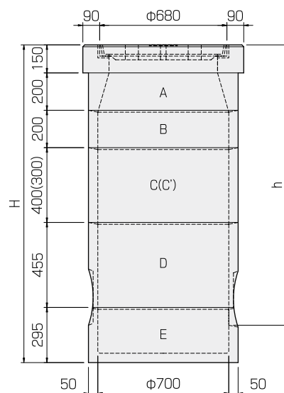
雨水樹(TMR70)
