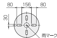
雨水枡蓋
