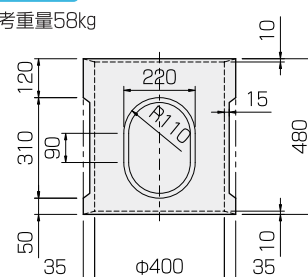
側塊B
