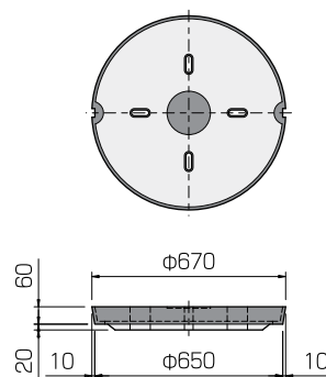
雨水樹蓋
