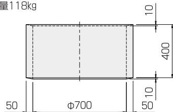
側塊C
