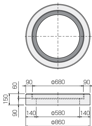
縁塊
