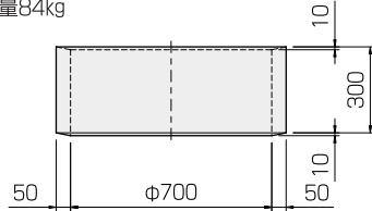
側塊C'
