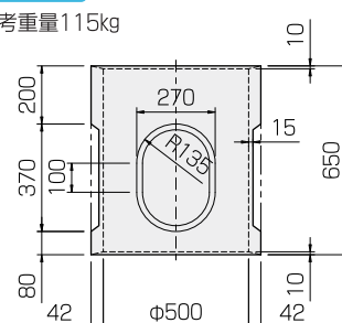
側塊B
