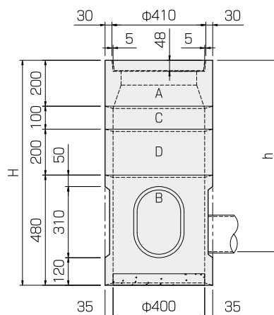
雨水枡(TMR40)
