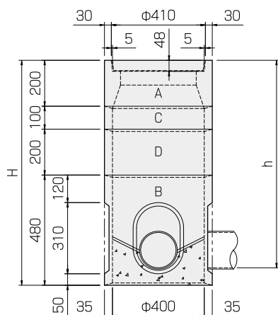
汚水枡(TMS40)
