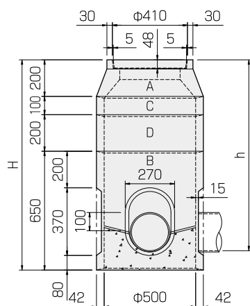
汚水枡(TMS50)
