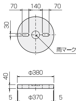
雨水桷蓋
