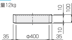
側塊C
