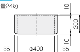
側塊D
