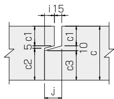
継手詳細図
