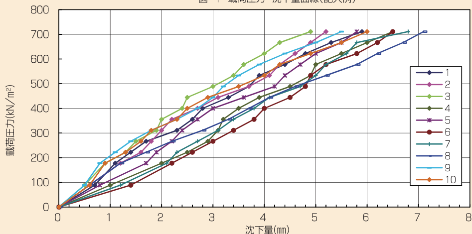
図-1 載荷圧力-沈下量曲線(記入例)
