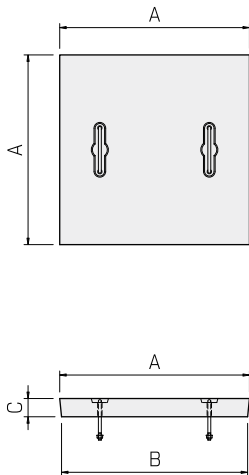
C型蓋
