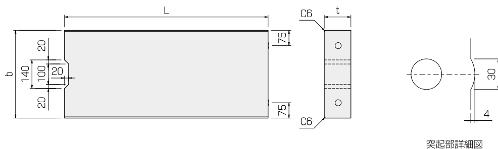
突起部詳細図
