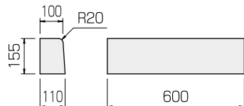
歩車道境界ブロック E-10
