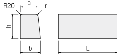
両面R
