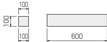
歩車道境界ブロック E-10
