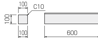
地先境界ブロック CE-AM
