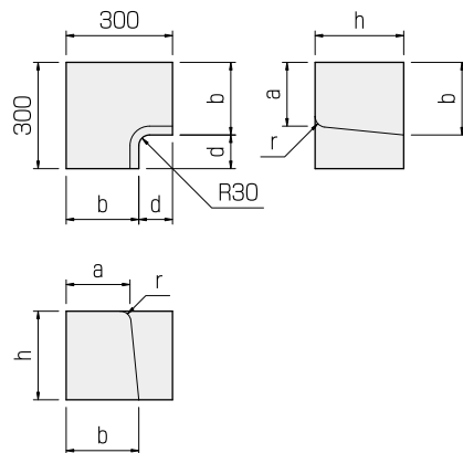
逆コーナー
