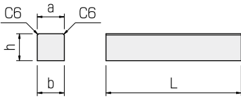
両面取り
